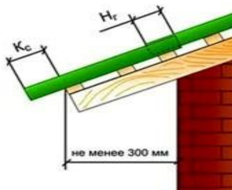
Рис. 1 Карниз кровли
